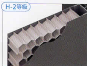
H-2等級 水酸化アルミ紙ハニカム構造 (断熱性能 H-2等級 U値 \leq 4.07W/(m^2 \cdot K) )
